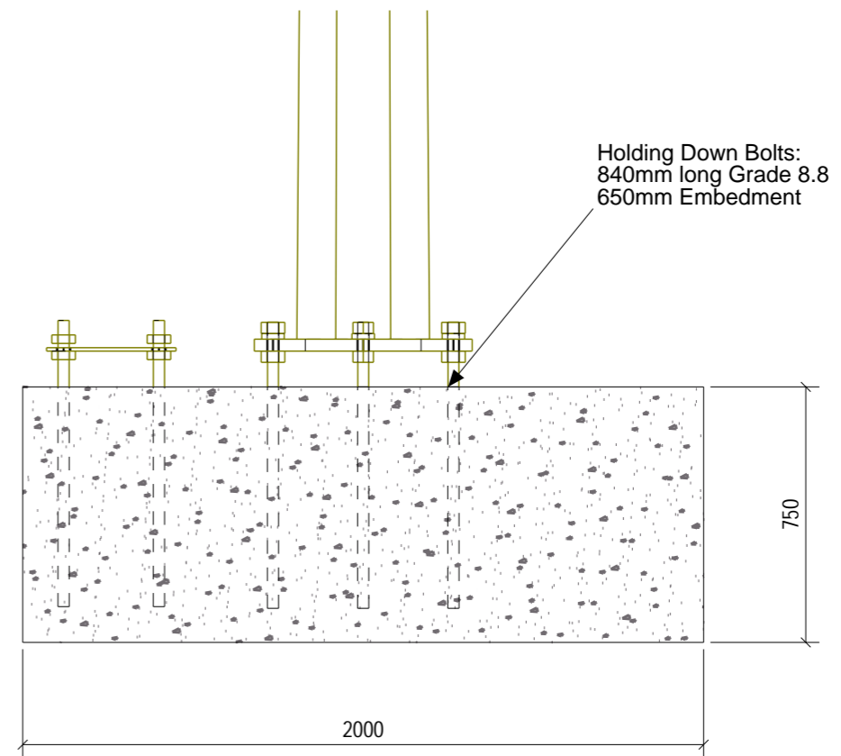
Section A-A 1:20
